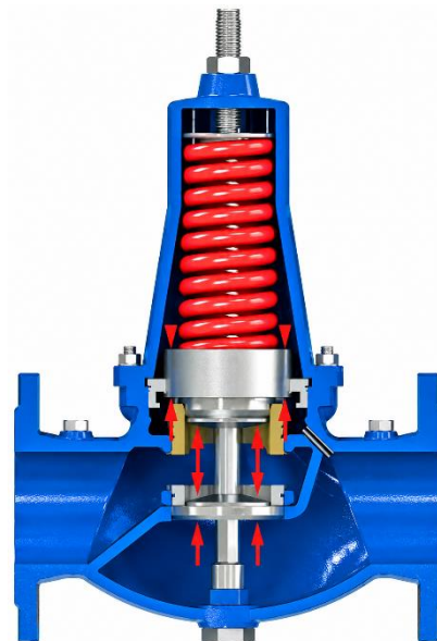
Vanne fermée (conditions statiques)
