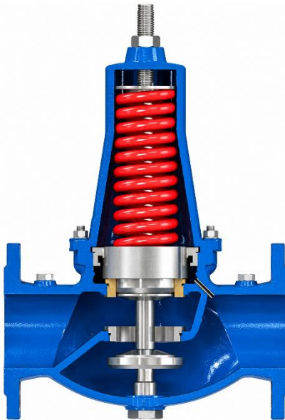
Vanne normalement ouverte
