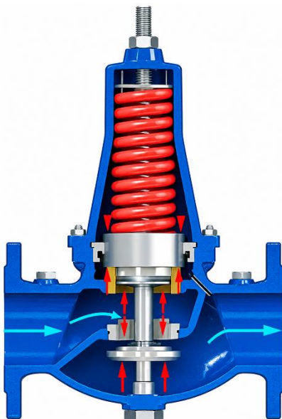
Vanne en régulation
