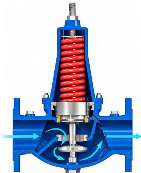
Vanne complètement ouverte
